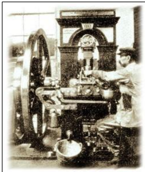
La primera máquina-herramienta fabricada en España: la prensa tipo Thonelier, construida por "La Maquinista Terrestre y Marítima" en 1863 para la Casa de la Moneda de Madrid. Fabricó las primeras pesetas, ahora desaparecidas.
