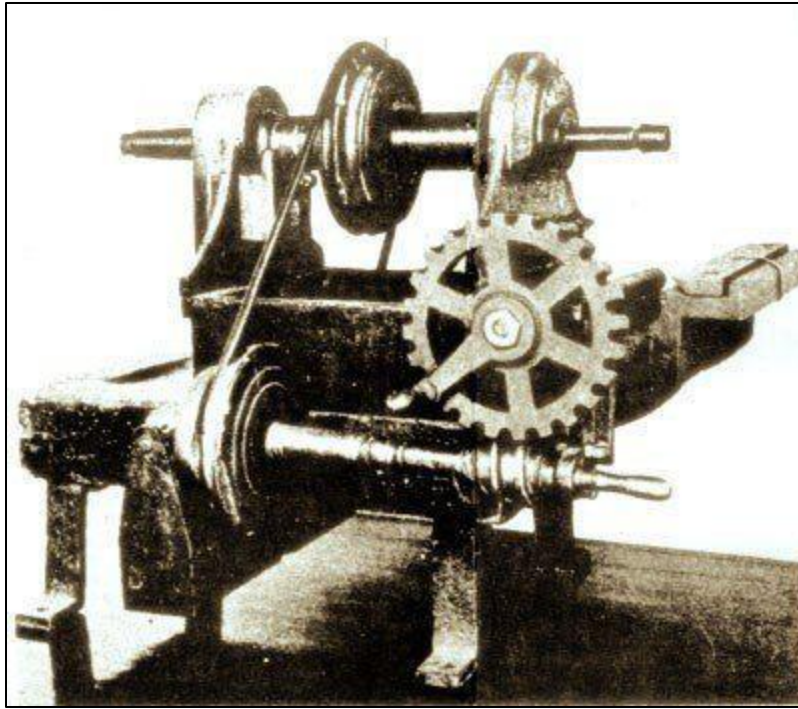
Co de Whitney, construida en 1818 para fabricar gran cantidad de fusiles en serie durante la guerra de la independencia americana. Destacaba un eje sinfín que se podía embragar y desembragar sobre una corona dentada alojada en el husillo del carro.
