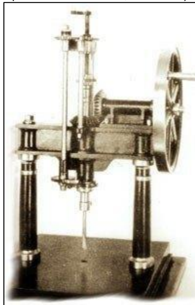
Taladro de sobremesa totalmente metálico, con giro de eje porta brocas accionado a mano o por transmisión fabricado por Nasmyth en 1938 (Science Museum, Londres).
