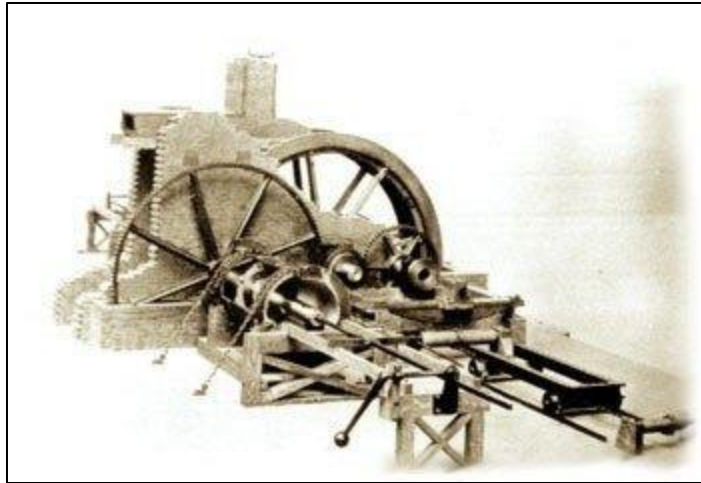
Mandrinadora de J. Wilkinson accionada por rueda hidráulica, fabricada en 1775 por encargo de James Watt. Se consiguió una precisión “del espesor de una moneda de seis peniques en un diámetro de 72 pulgadas” (Science Museum, Londres).
