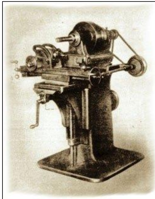
Primera fresadora universal, fabricada por Joseph R. Brown en 1862. Estaba equipada con divisor, consola con desplazamiento vertical, curso transversal y avance automático de la mesa longitudinal con la aplicación de la transmisión Cardan
